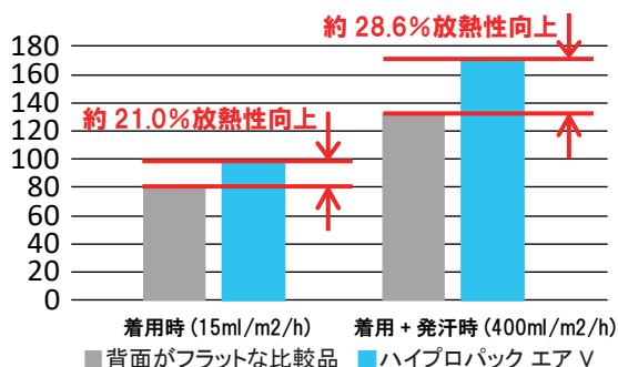
（図1）背面2部位の平均放熱量 [W/m 2 ]
